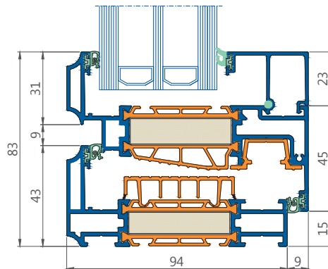
verticale doorsnede
