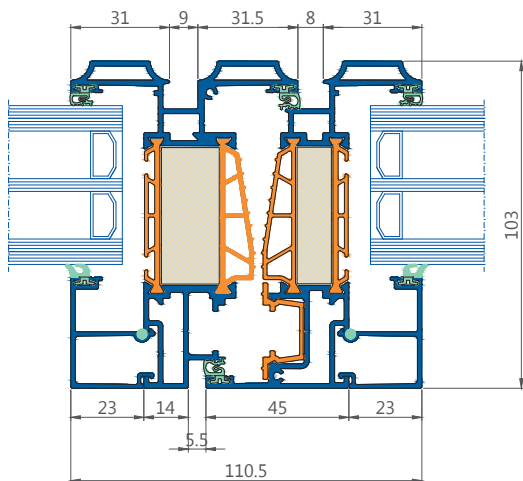
horizontale doorsnede
