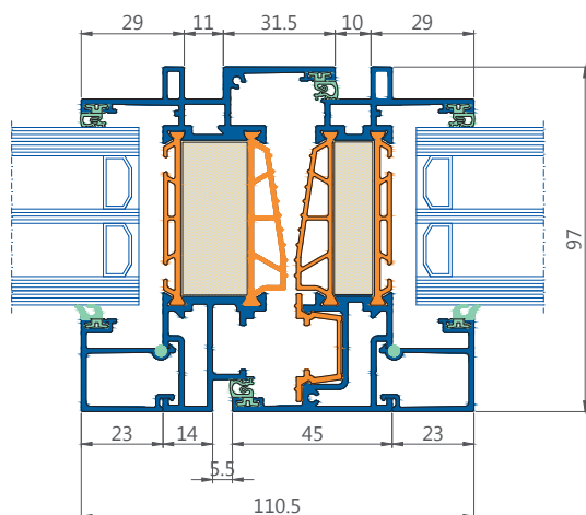
horizontale doorsnede
