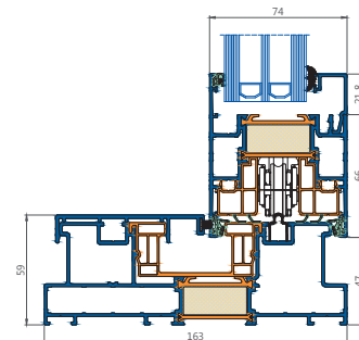
verticale doorsnede duorail
