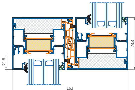
horizontale doorsnede
